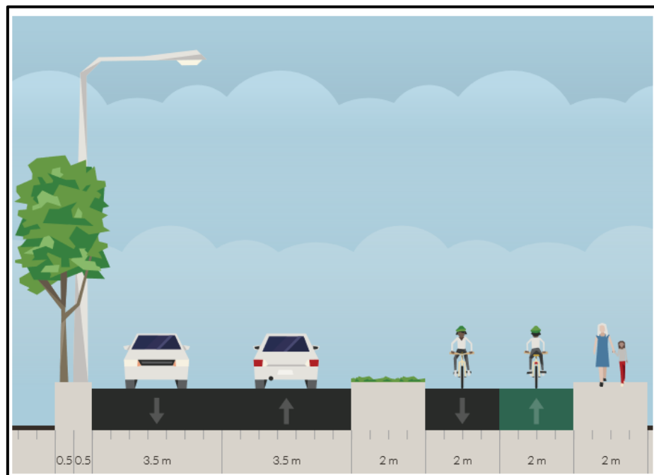
Figur 2: Snitt i Hogsnesbakken.
